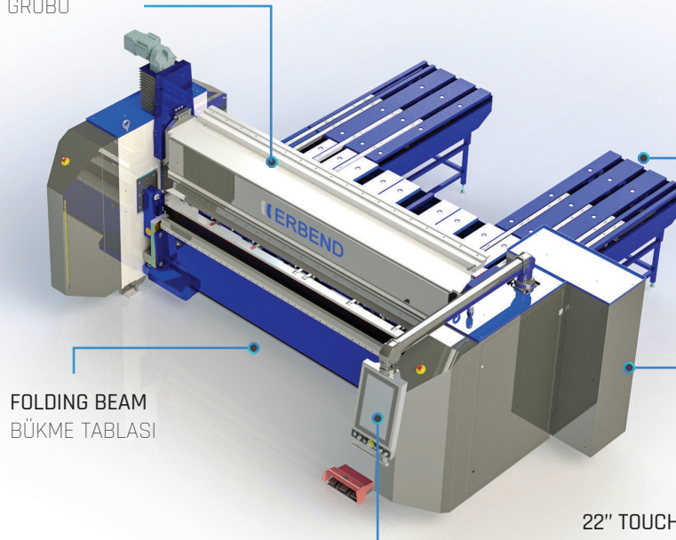
ROTATING COMBI UPPER BEAM GROUP DÖNERLİ ÜST TABLA GRUBU
